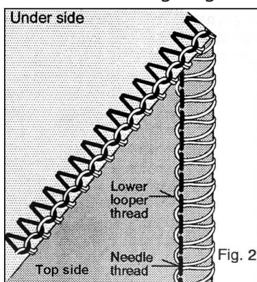
Nadelfadenspannung verringern
