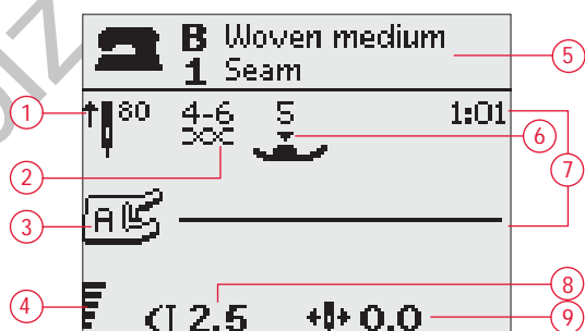
Běžný šicí mód, Rovný steh
