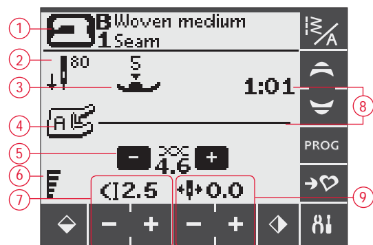
Běžný šicí mód, Rovný steh
